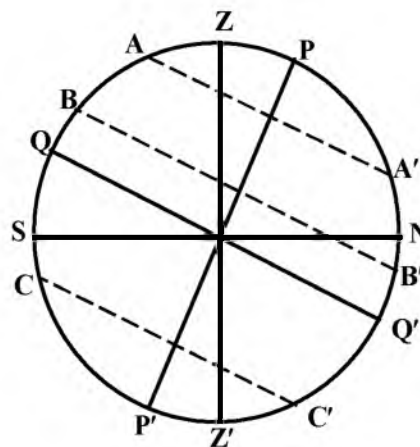
Рис.2. Проекція добових паралелей на площину небесного меридіану
