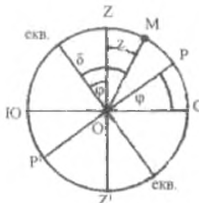
Рис.4. Верхня кульмінація на північ від зеніту
