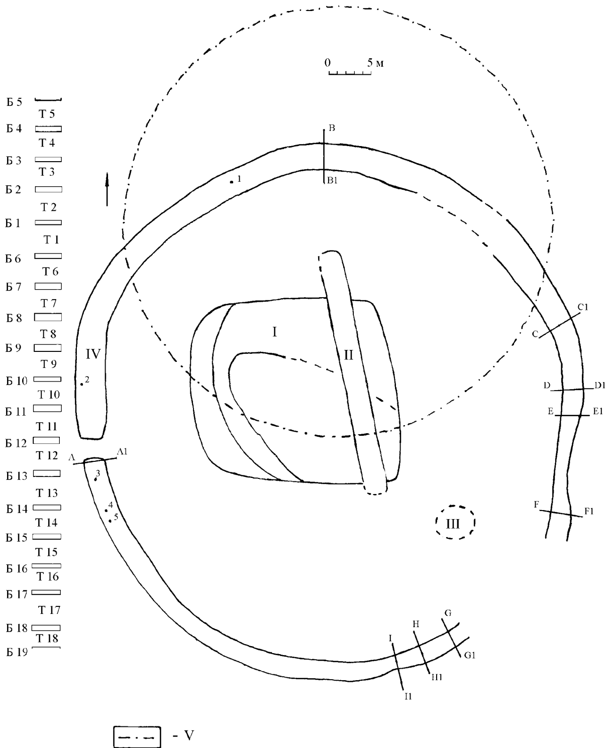
Рис. 10. Мельгуновский курган, плаи (раскопки 1990 г.). I – прямоугольная яма и II – прорезающая ее траншея в центральной части; III – яма в юго-восточном секторе; IV – ров с перемычкой на западе; V – первоначально предполагаемые контуры кургана. Б – бровка; Т – траншея. 1 – фрагмент стенки амфоры, 2 – обломок ножки амфоры, 3 – фрагмент лепного сосуда, 4 – гранитные терочник и часть грузила, 5 – кремьень.
