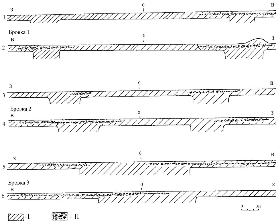
Рис. 11. Профили бровок Мельгуиовского кургаиа (раскопки 1990 г.). 1, 2 – бровка 1, южный и северный профили. 3, 4 – бровка 2, южный и северный профили. 5, 6 – бровка 3, южный и северный профили.
